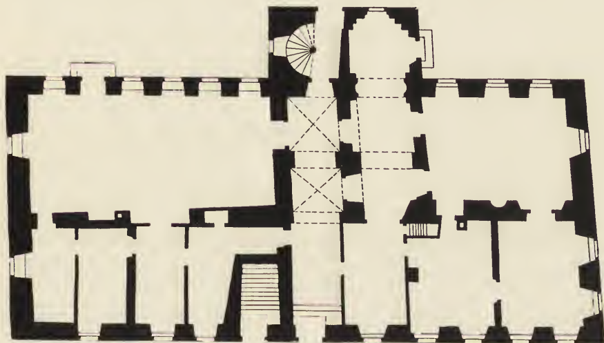
Fig. 37. Döbeln. Rathhaus, Grundriss des Erdgeschosses.
